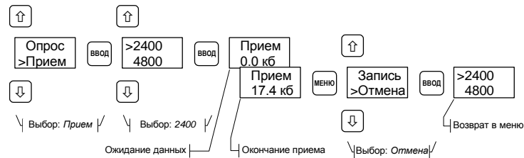
Рисунок 5.6 Режим Прием . Завершение чтения без запоминания данных
